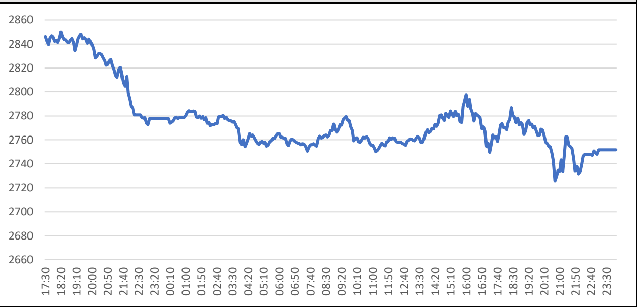
S&P 500 Future
